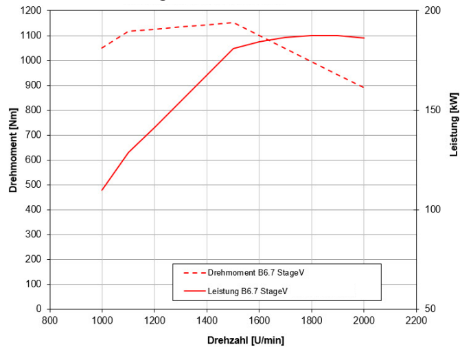
Leistung und Drehmoment PB 100
